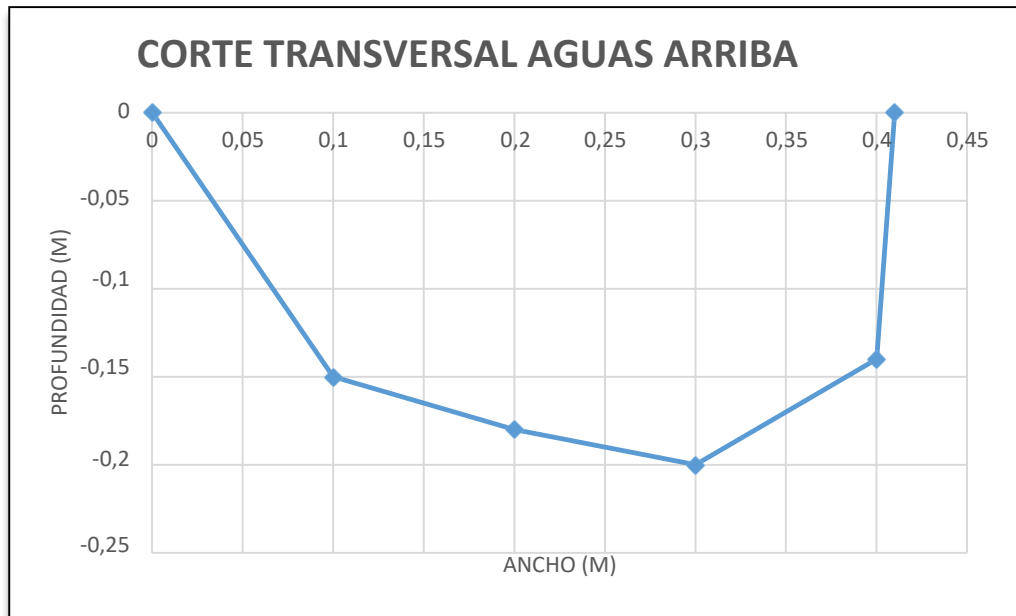
Gráfica 1. Corte transversal aguas arriba
