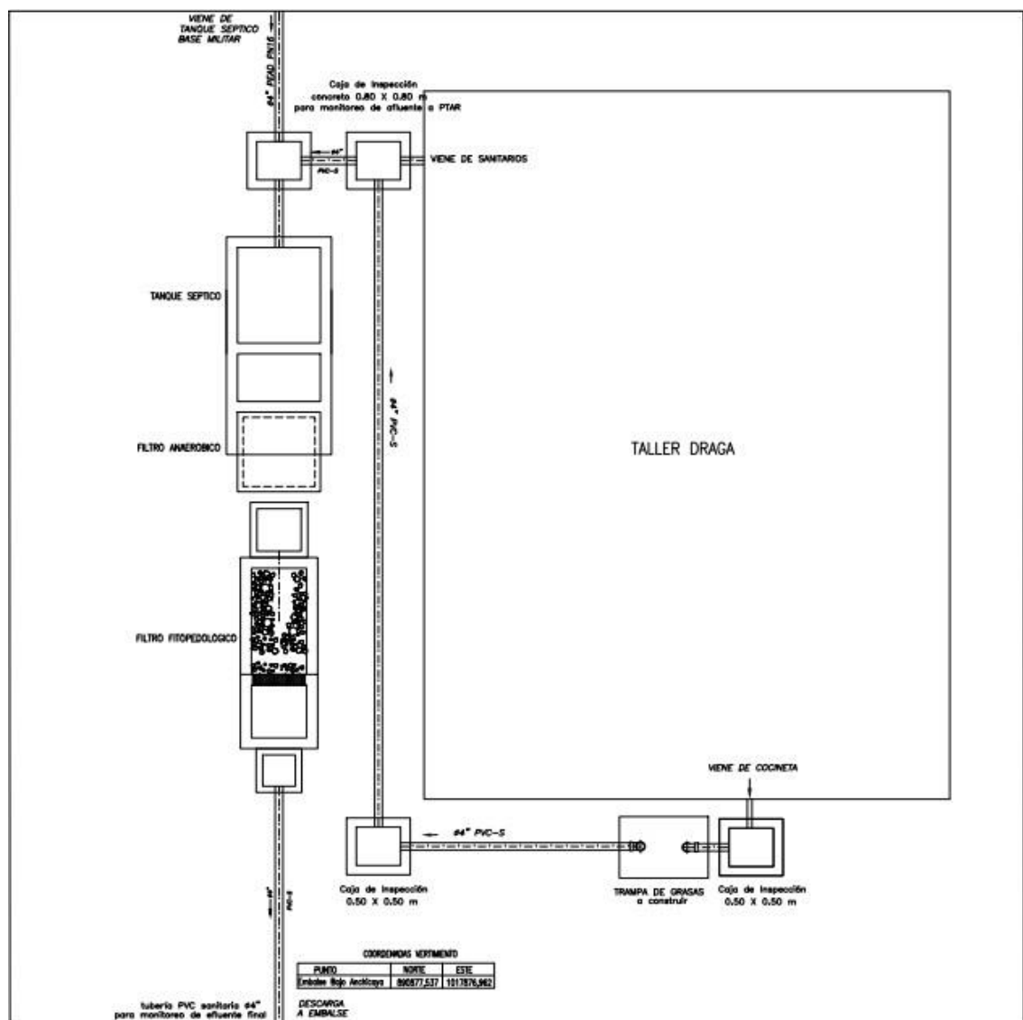
Figura 1. Diagrama del Sistema de Tratamiento. Fuente: Celsia Colombia S.A. E.S.P.-
