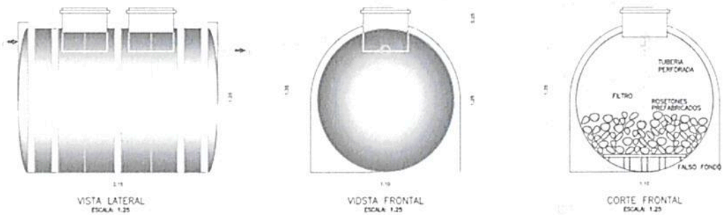
SISTEMA SEPTICO INTEGRADO DE 2000Lts
