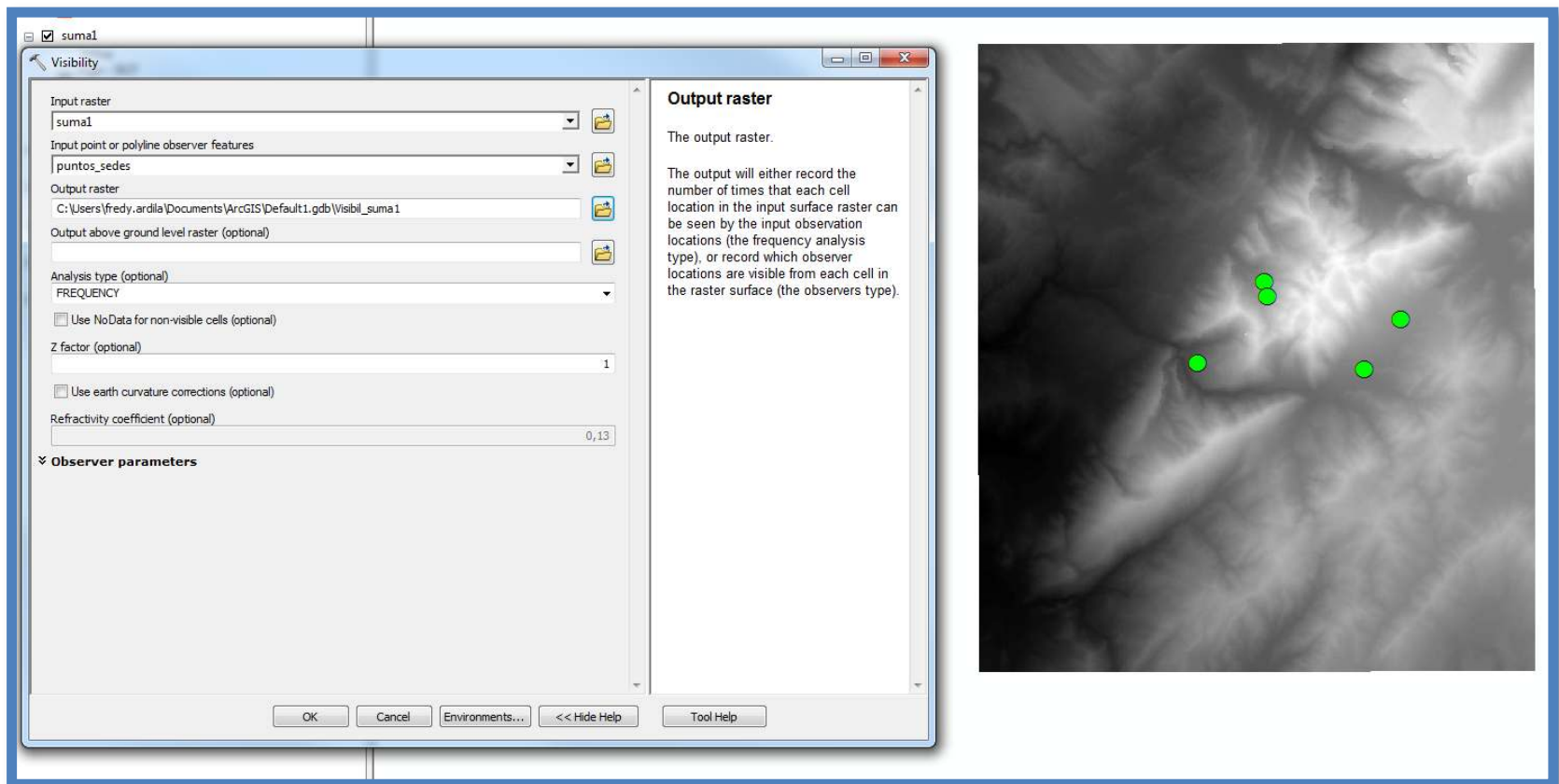
Ilustración 13 cálculo de visibilidad tipo punto con visibility
