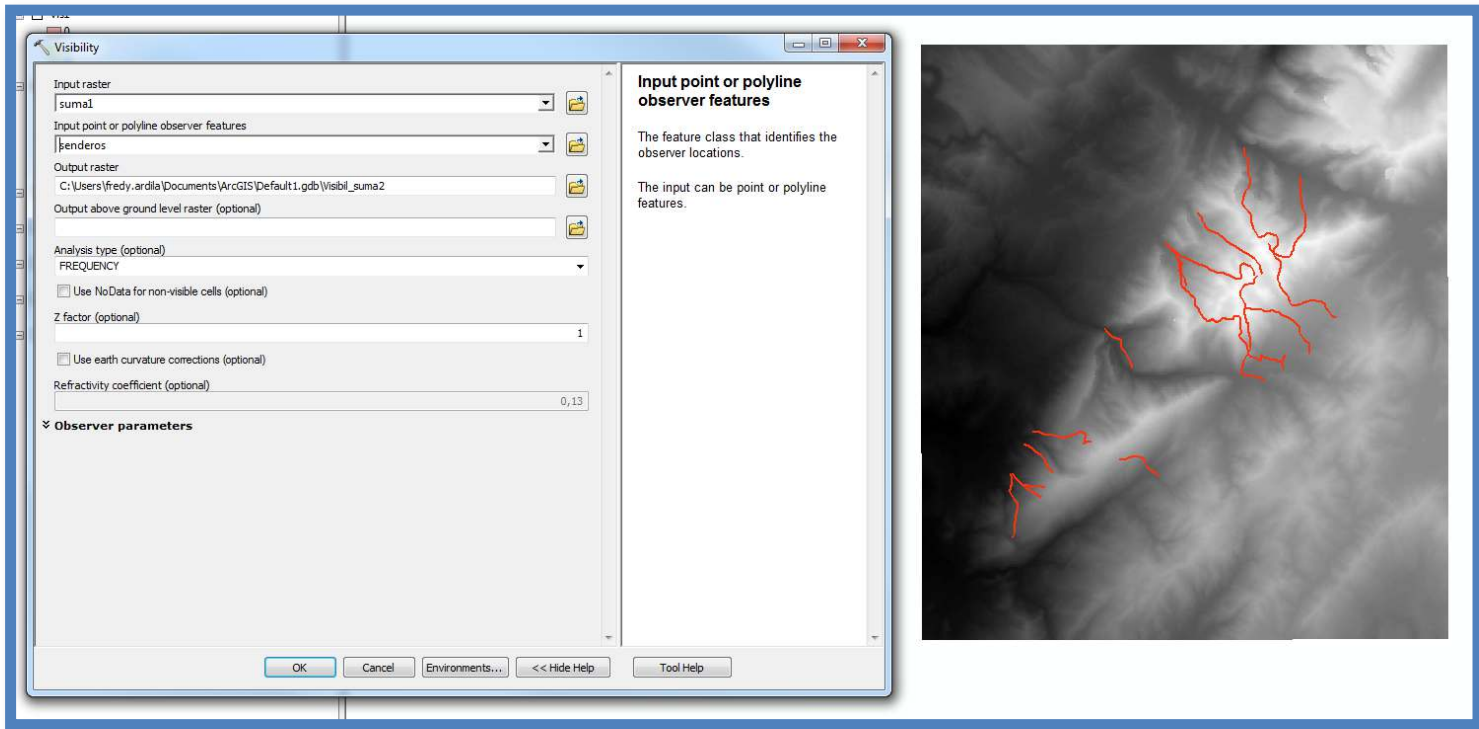
Ilustración 16 cálculo de visibilidad tipo línea con visibility
