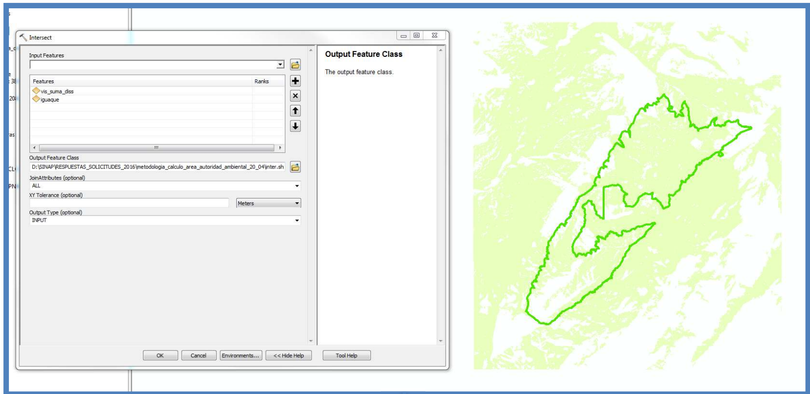
Ilustración 25 selección de área efectiva al interior del área protegida
