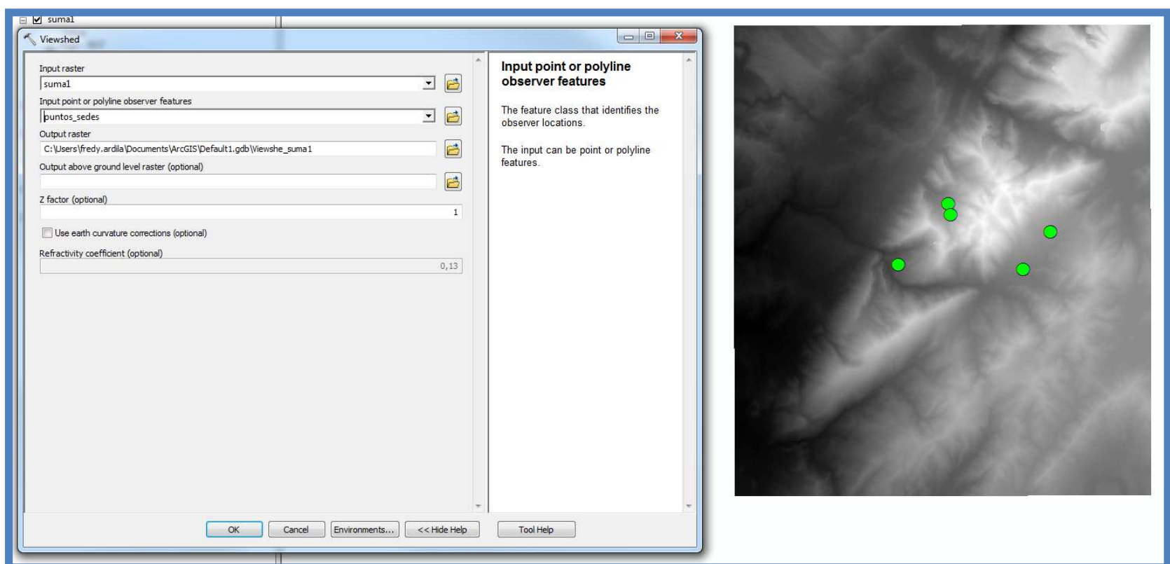
Ilustración 14 cálculo de visibilidad tipo punto con viewshed
