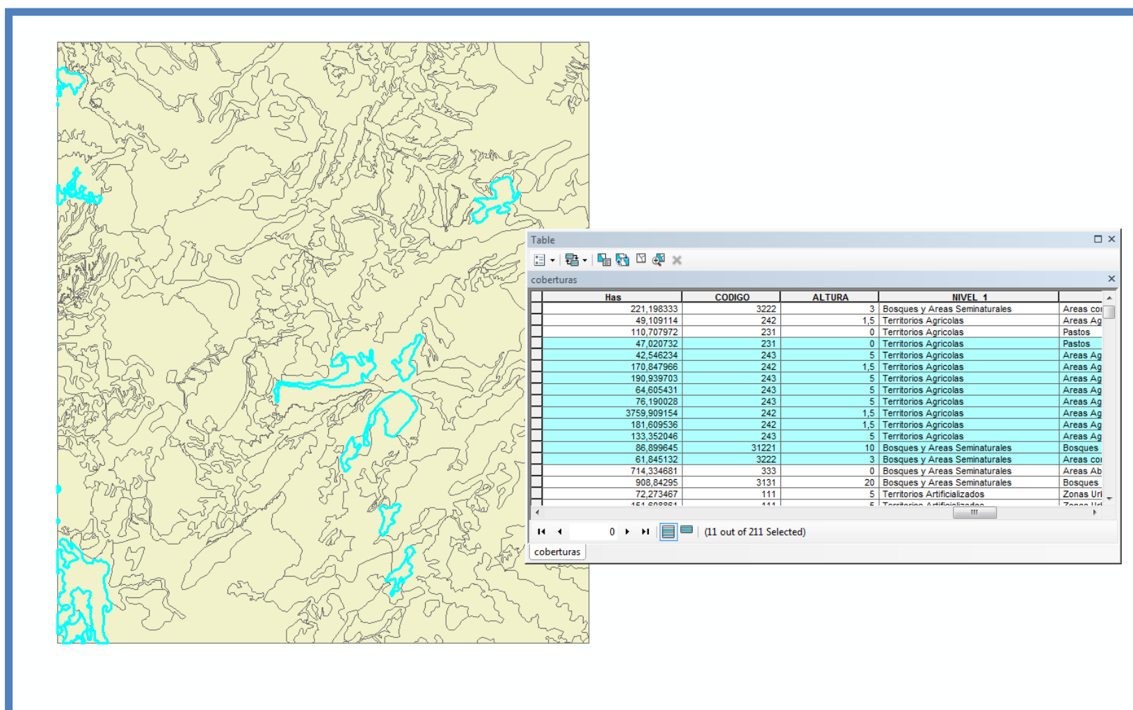
Ilustración 9 coberturas vegetales con alturas incorporadas
