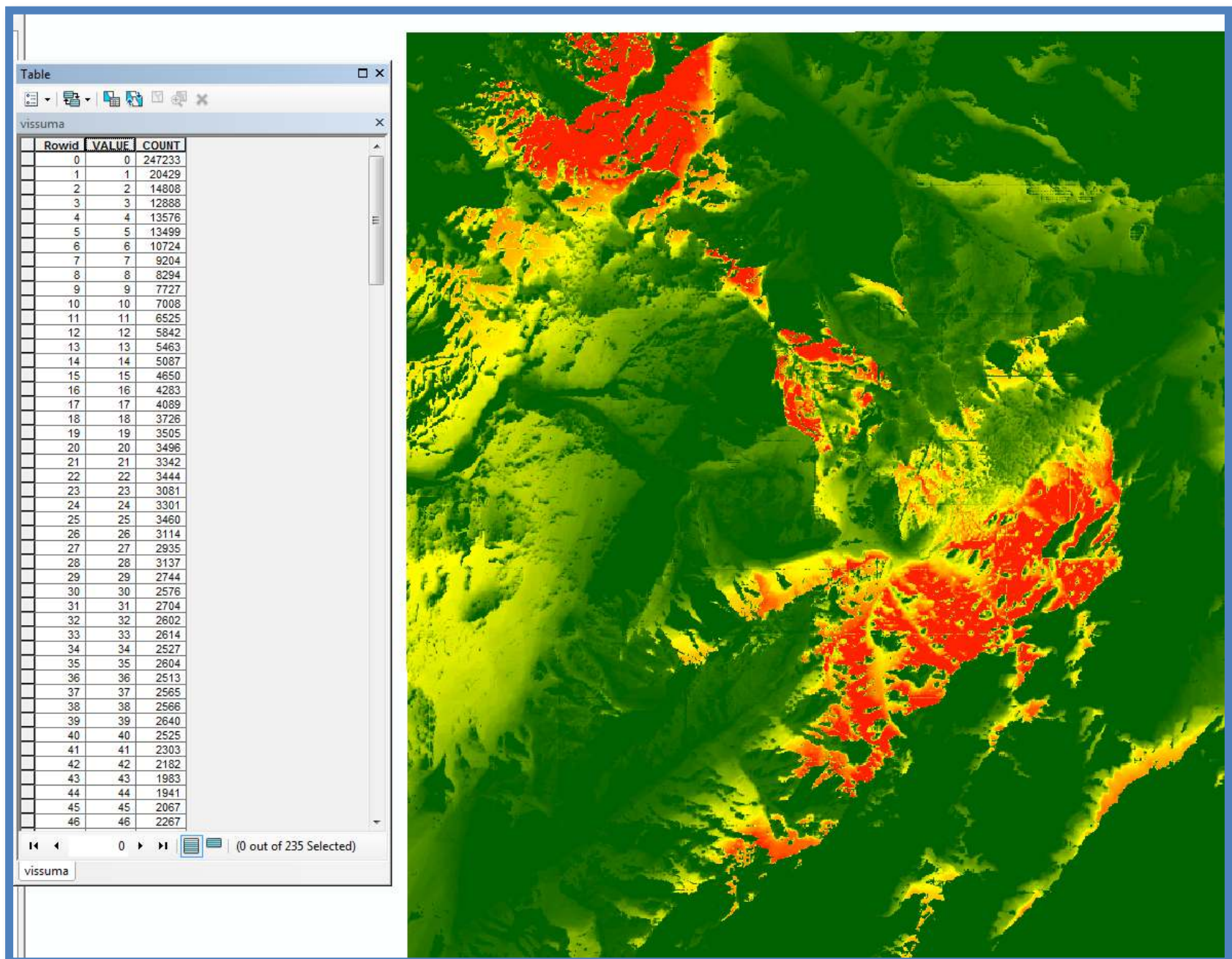
Ilustración 20 raster del área de trabajo con área visualizada desde puntos y senderos de PVC
