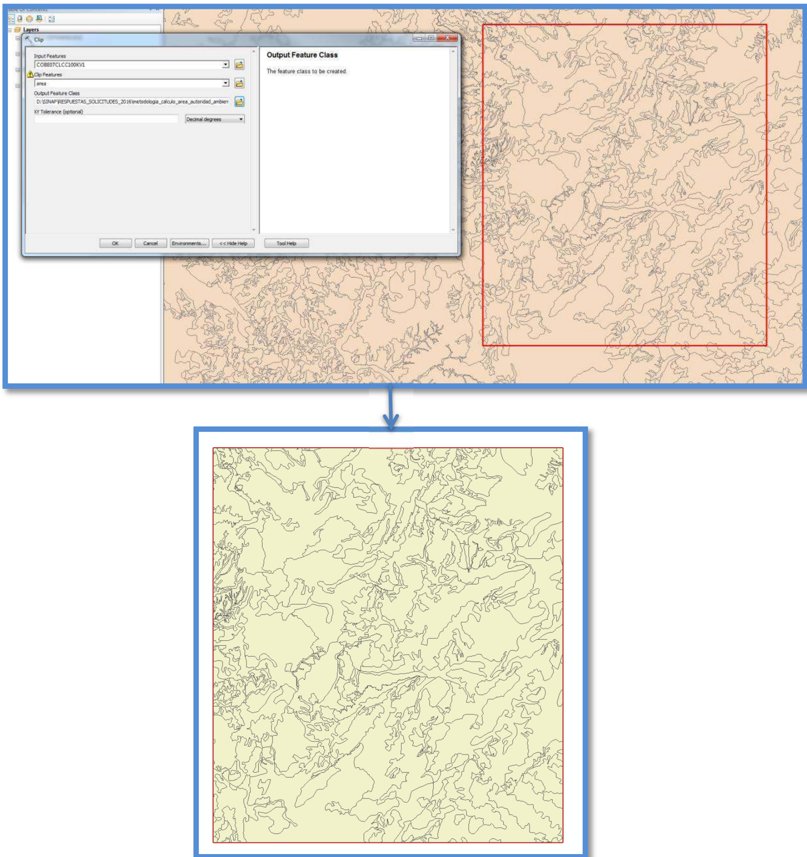
Ilustración 3 ejemplo de clip de coberturas de la tierra al área de trabajo
