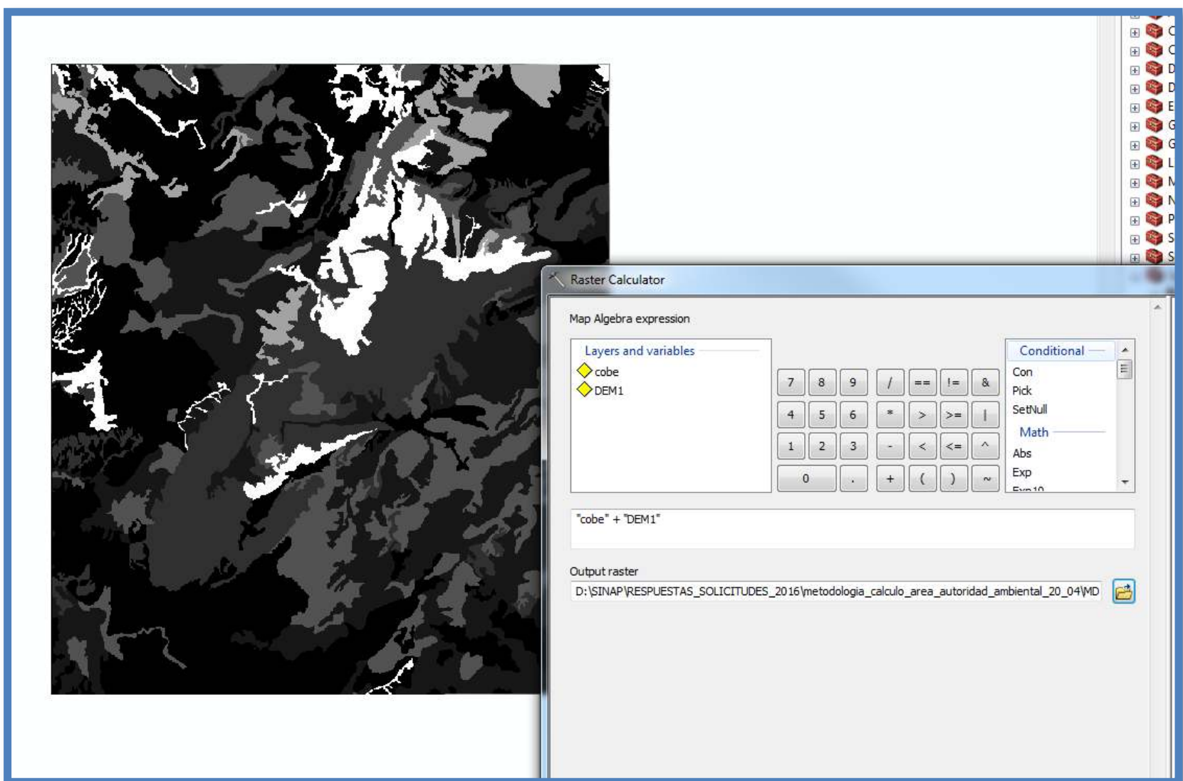
Ilustración 11 herramienta de suma de raster DEM y raster de coberturas vegetales con altura
