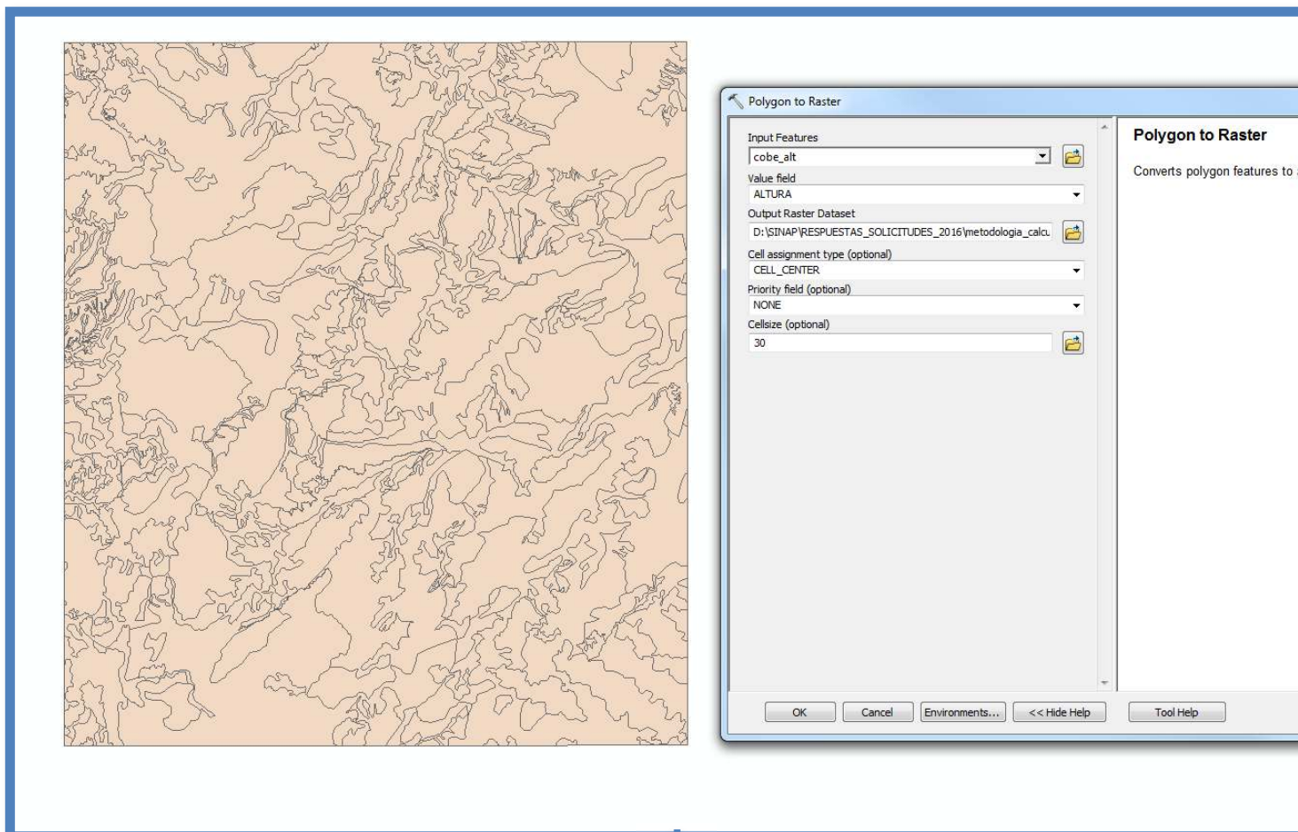
Ilustración 10 rasterización de capa de coberturas vegetales con alturas
