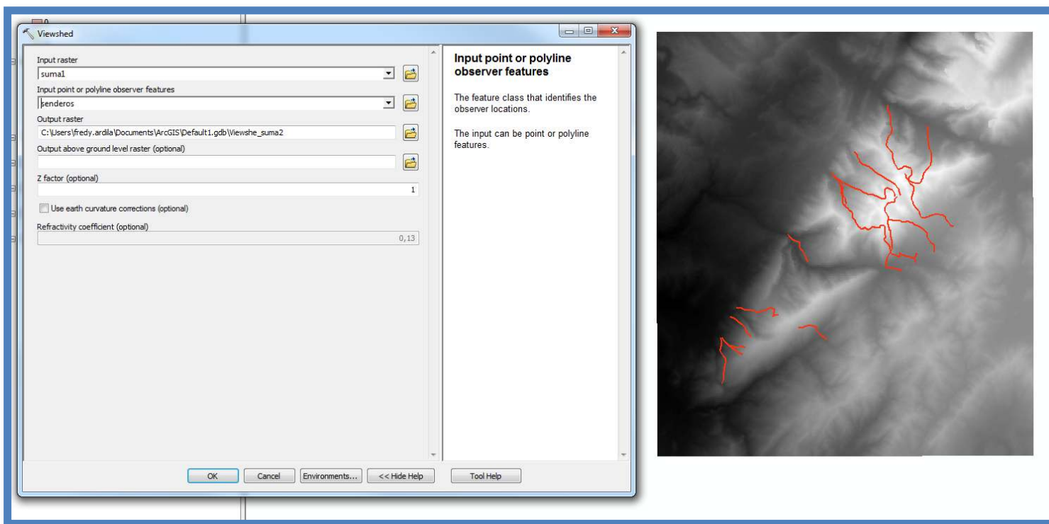
Ilustración 17 cálculo de visibilidad tipo línea con viewshed
