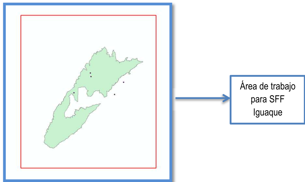
Ilustración 2 ejemplo de área de trabajo definida para SFF Iguaque
