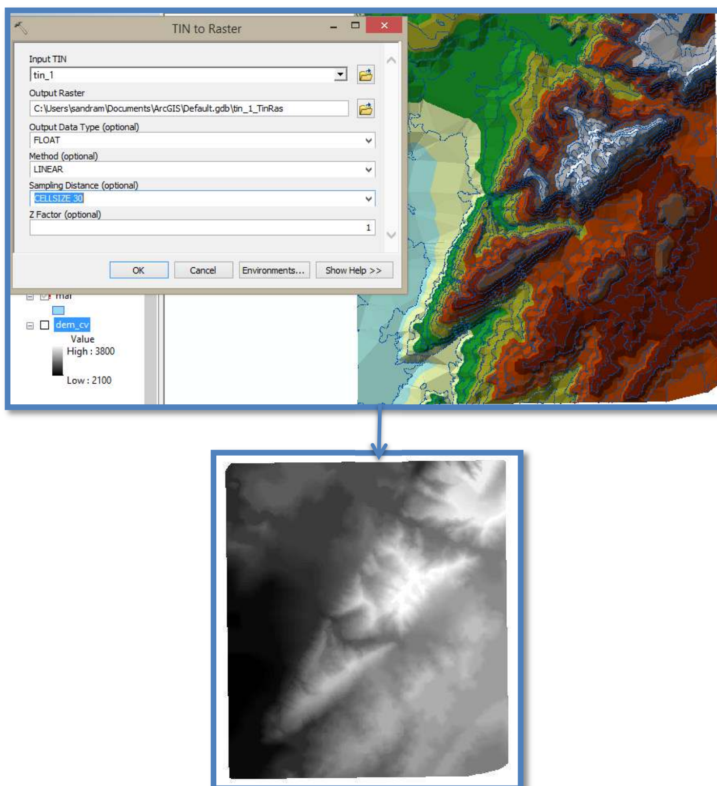
Ilustración 7 creación del DEM a partir del TIN
