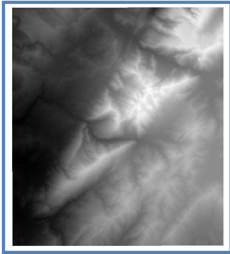
Ilustración 12 archivo raster con alturas del DEM y coberturas vegetales
