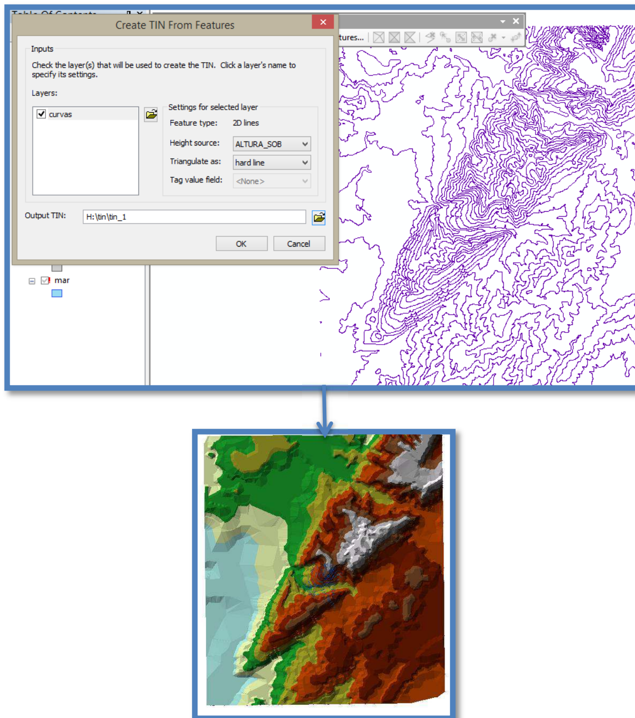
Ilustración 6 creación del TIN a partir de las curvas de nivel
