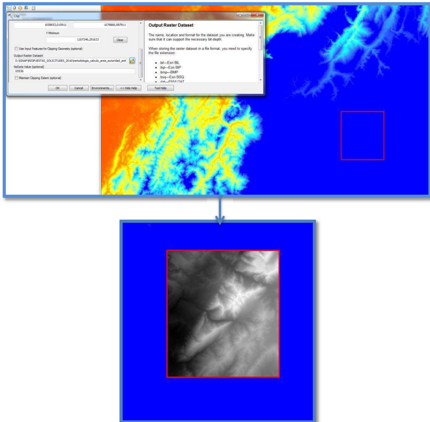
Ilustración 5 ejemplo de clip de DEM (raster) al área de trabajo
