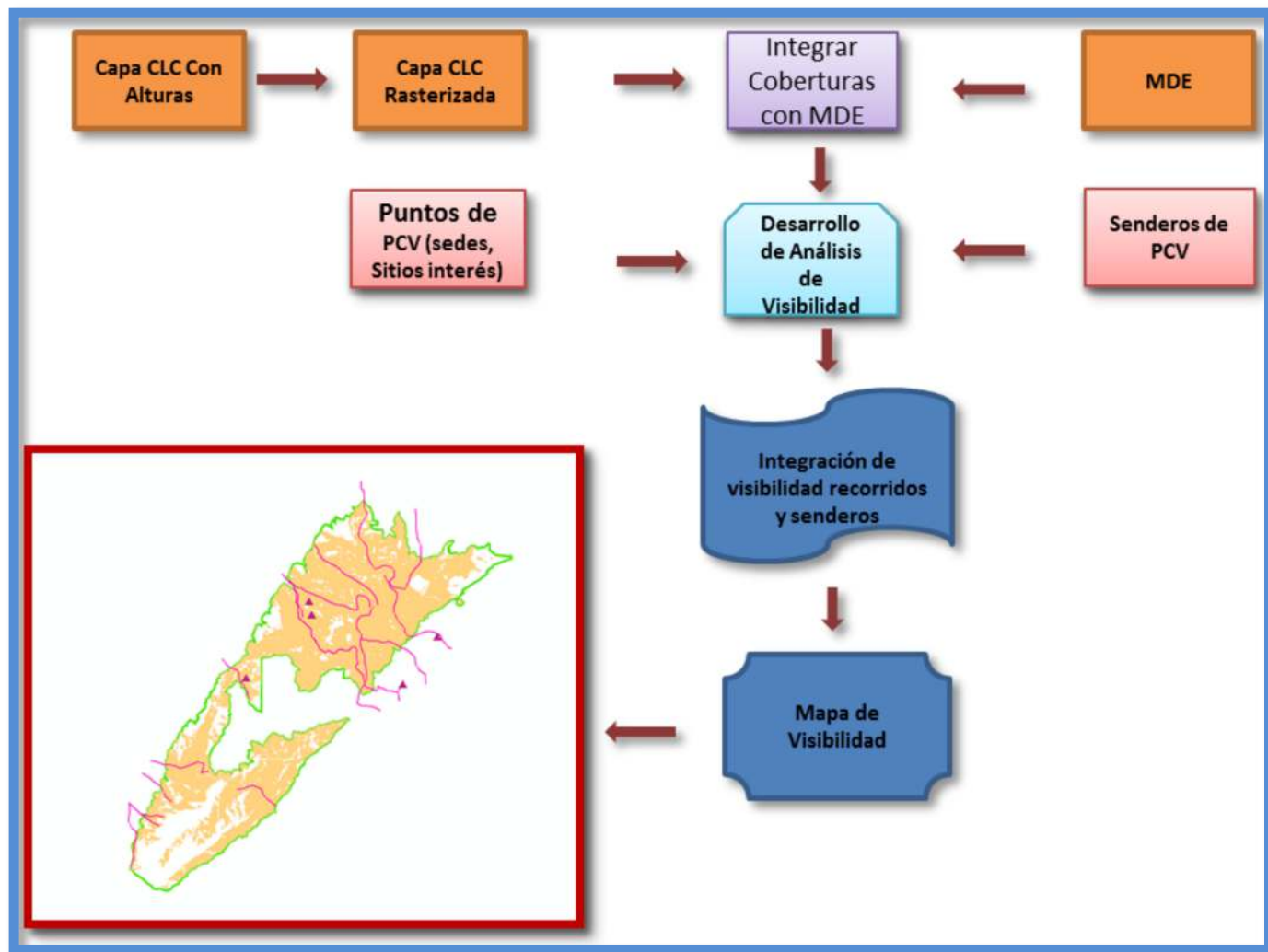
Ilustración 1 diagrama general de metodología establecida
