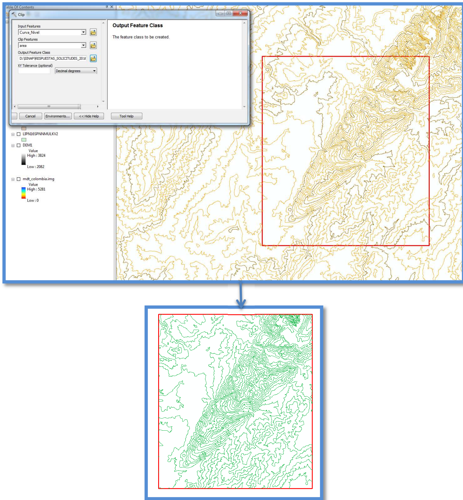
Ilustración 4 ejemplo de clip de curvas de nivel al área de trabajo
